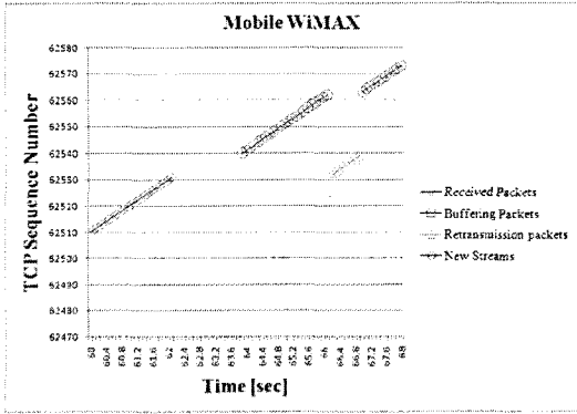
그림 10. Mobile WiMAX의 TCP 순서 번호
