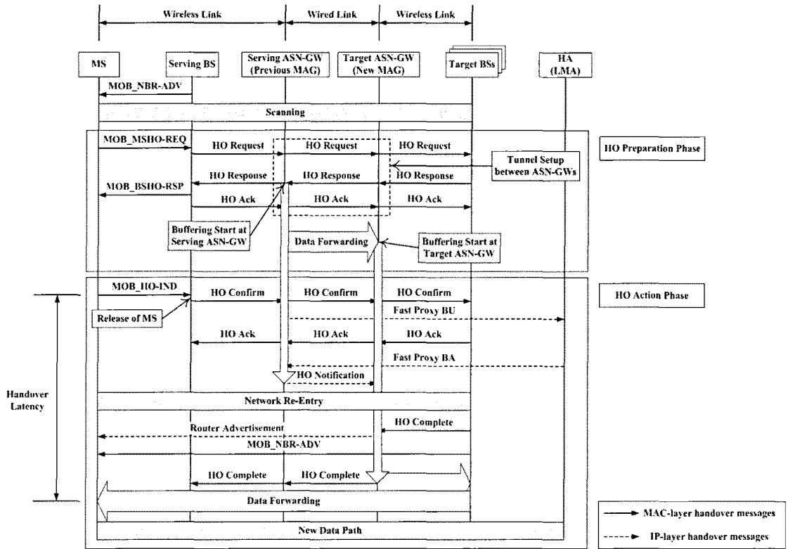
그림 4. Mobile WiMAX 기반의 무선 매쉬 네트워크를 위한 PMIP 기반의 고속 3계층 핸드오버
