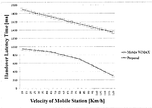
그림 14. 단말 속도 변화에 따른 핸드오버 지연
