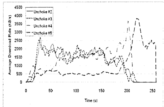
그림 5. 2개 호스트씩 무리를 지은 4개의 그룹이 각각 2개 3개 4개 5개의 unchoke 개수를 가질 때 Average Download Rate
