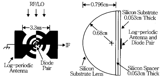
(a) Log-periodic 안테나 (b) Si 렌즈 구조
