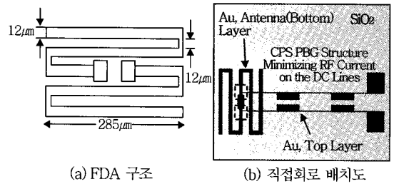
(그림 14) Planar Wideband 80~200GHz Receiver[16]
