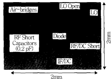
(b) 직접회로 배치도
