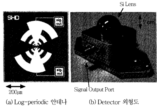
(a) Log-periodic 안테나 (b) Detector 외형도
