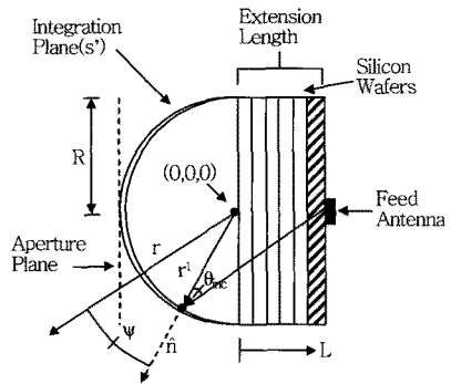
(그림 5) Extended Hemispherical Lens[8]
