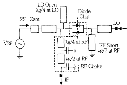
(a) SHM 회로구성도
