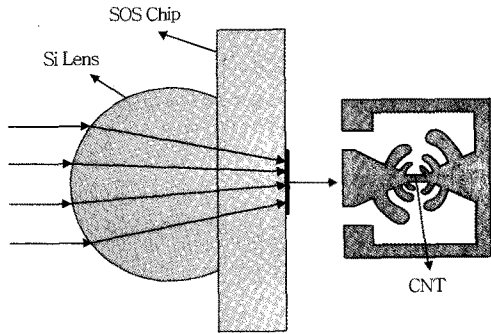
(그림 4) Lens-Antenna Quasi-Optical Coupling Configuration[7]
