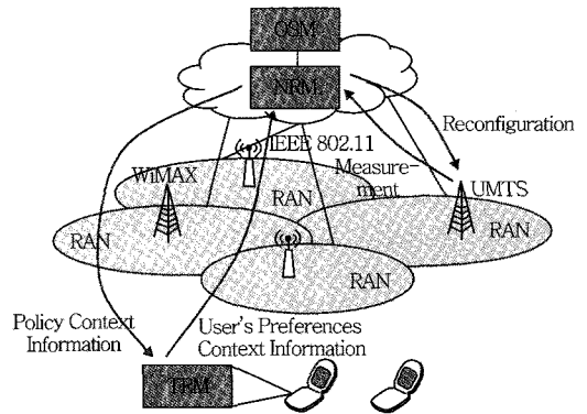
(그림 4) IEEE P1900.4에서의 CWN 환경
