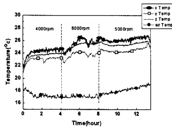
그림 5. 장시간 가공중 발생하는 가공축의 온도 변화
