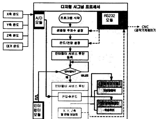
그림 8. 보정모델(선형회귀모델 및 신경회로망모델)이 탑재된 열변형 보상장치 내부구성도
