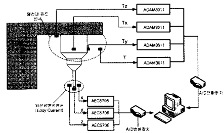
그림 1. 기본적인 열변형 데이터 취득 실험 구성도
