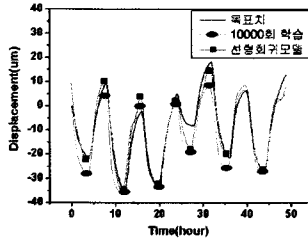
그림 9. 보정모델의 열변형 예측치의 신뢰도 확인
