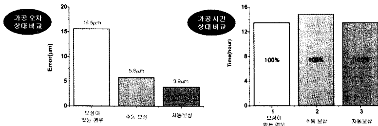
그림 13. 가공 및 보정의 실제 실험
