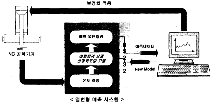
그림 2. 가공중 실시간 보정을 위한 열변형 보상 실험장치 구성도
