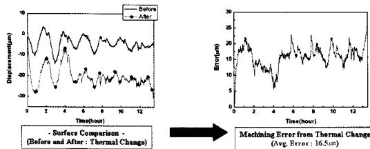
그림 6. 장시간 가공중 온도변화에 따른 열변형 평균 오차 추출
