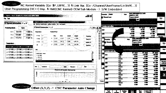
그림 11. 실시간 열변형 보상을 위한 CNC에서의 기계원점 자율보정
