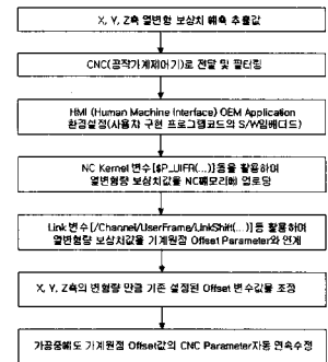
그림 10. 실시간 열변형 보정을 위한 임베디드 보상장치와 CNC와의 연계도
