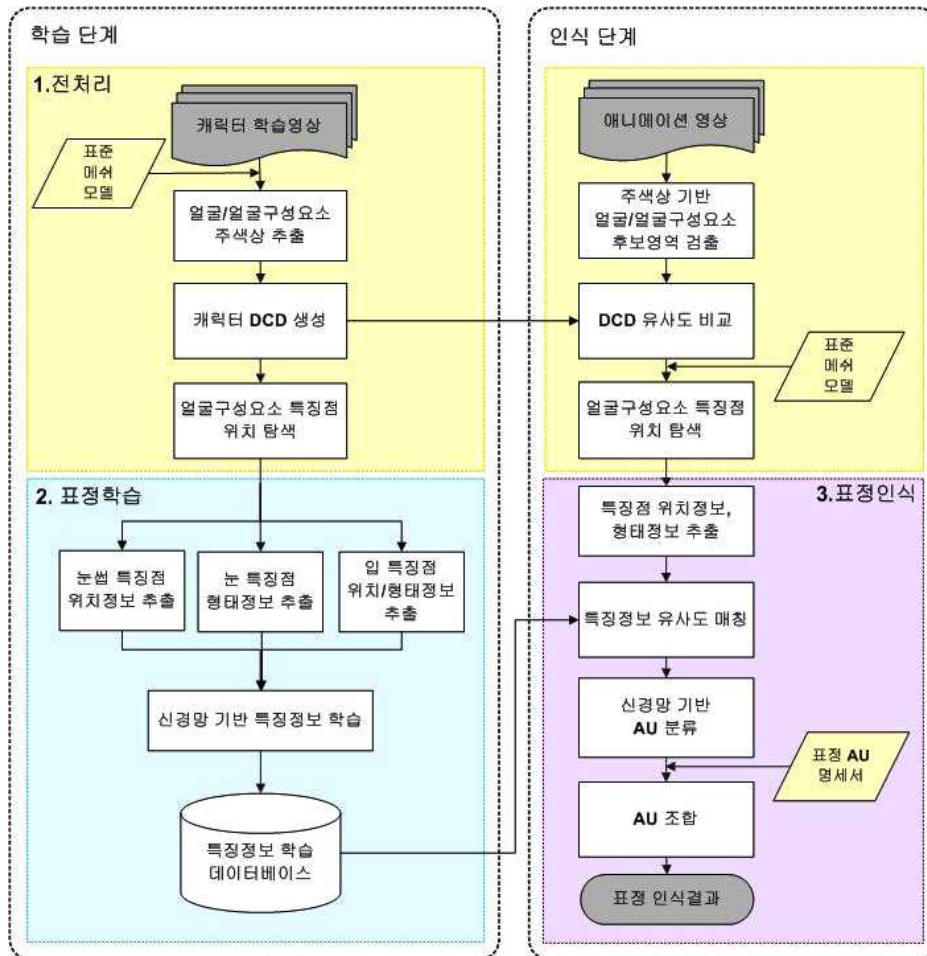
(그림 1) 전체 개요도
