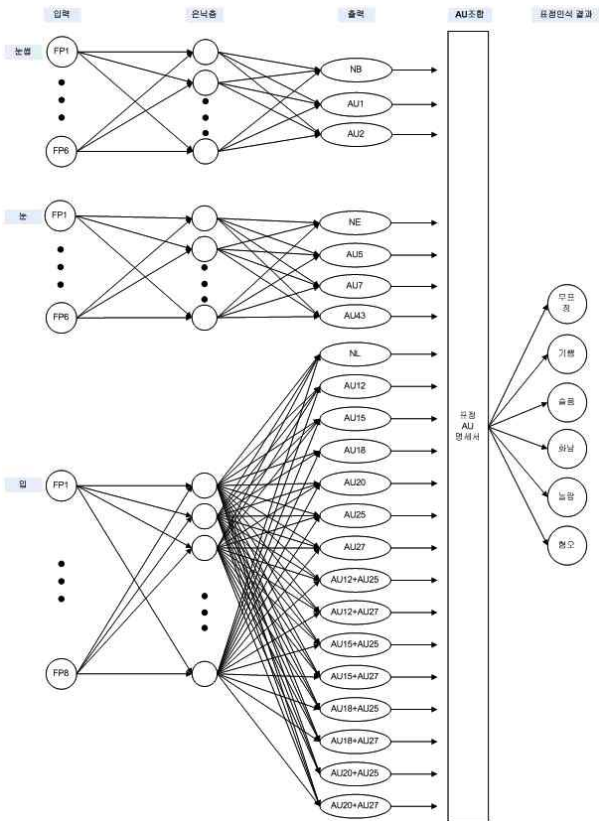
(그림 9) 표정인식을 위한 신경망
