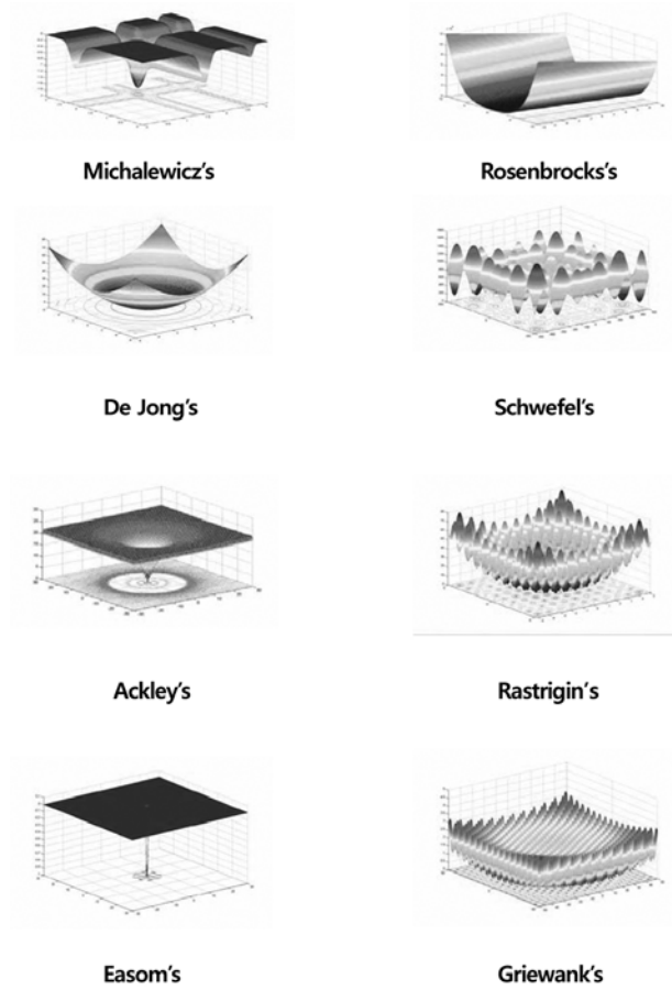
(그림 1) 실험에 사용한 벤치마킹 함수들의 2차원 도메인 표현
