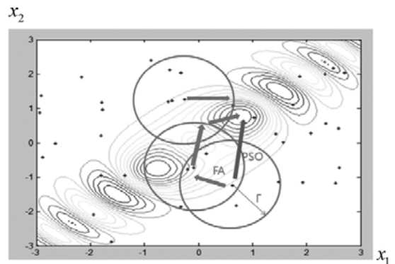
(그림 3) FA와 PSO의 각 입자의 이동방법 비교
