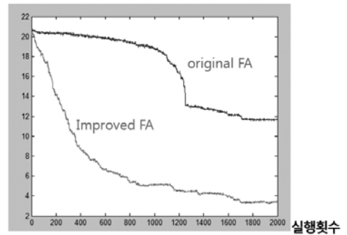
(그림 4) Ackley의 함수에 대한 FA와 Improved FA의 비교
