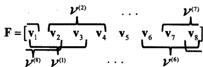
그림 2. N_i = 4, B = 3 인 경우, 코드북과 직교 부분집합
