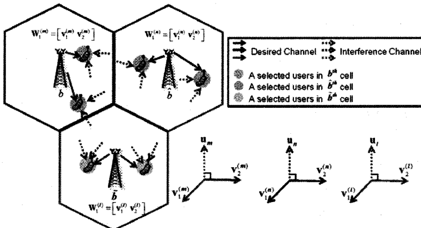
그림 4. N_i = 3, \eta = 1 일 때, 두 기지국 사이의 협력적 스케줄링 및 빔형성 기법
