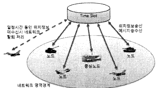
그림 2. 메시지를 송수신하는 노드의 네트워크 영역 이탈 Fig 2. Leaving the network for TX-RX node
