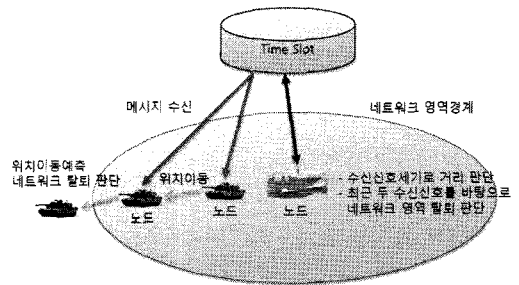
그림 4. RSSI 신호를 이용한 네트워크 영역 이탈 판단 Fig 4. Decision for node of leaving the network using RSSI signal
