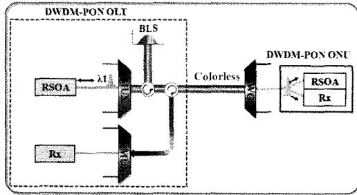
그림 5. RSOA 기반 DWDM-PON 링크 구조
