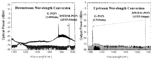
그림 11. 하이브리드 PON에서 파장변환 결과
