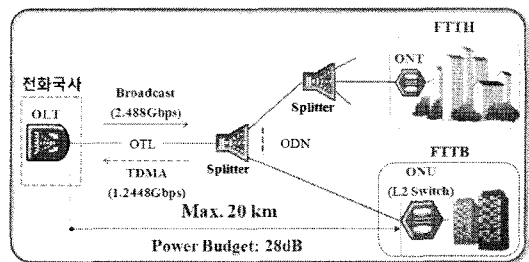
그림 1. 일반 G-PON 링크 구조
