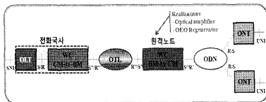
그림 3. G-PON 거리 확장 구조
