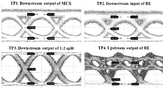
그림 9. DWDM-PON에서 측정된 Eye Pattern
