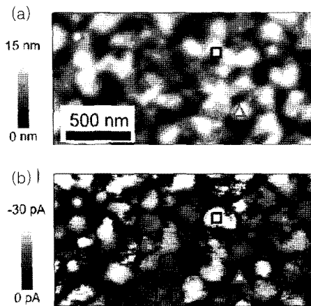
그림 6. P3MPV-PPV/PCBM(20:80 ratio) 필름의 AFM height image (a)와 광전류 이미지 (b). 광전류 측정에서 파장은 532 nm, 세기는 104 \text{ W m}^{-2} .
