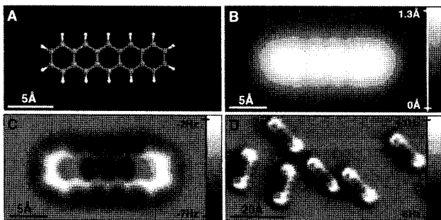
그림 1. (A) pentacene 분자 모형. (B) pentacene 분자의 STM image. (C, D) CO 분자로 흡착된 탐침을 이용하여 스캔한 pentacene 분자의 AFM image. 이 경우 pentacene 분자내의 다섯개의 benzene 링의 식별이 가능하다.
