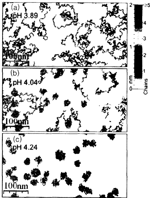
그림 8. 세가지 서로 다른 pH 영역에서의 poly(2-vinylpyridine) 고분자 형태 변화, pH가 증가함에 따라서 랜덤 코일 형태에서 compact coil 형태로 전이가 일어남.
