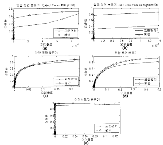
그림 8. 기존 방법과 제안한 방법을 사용하여 학습시킨 분류기들의 ROC 커브. (a) Caltech Faces 1999 (Front) 샘플을 사용한 얼굴 정면 분류기 평가 결과, (b) MIT CBCL Face Recognition Database 샘플을 사용한 얼굴 정면 분류기 평가 결과, (c) 차량 전면 분류기 평가 결과, (d) 차량 후면 분류기 평가 결과, (e) 야간 보행자 분류기 평가 결과.
