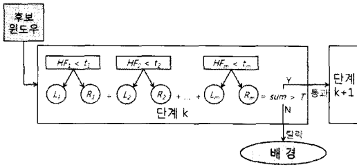
그림 4. 다단계 분류기의 각 단계의 구성.
