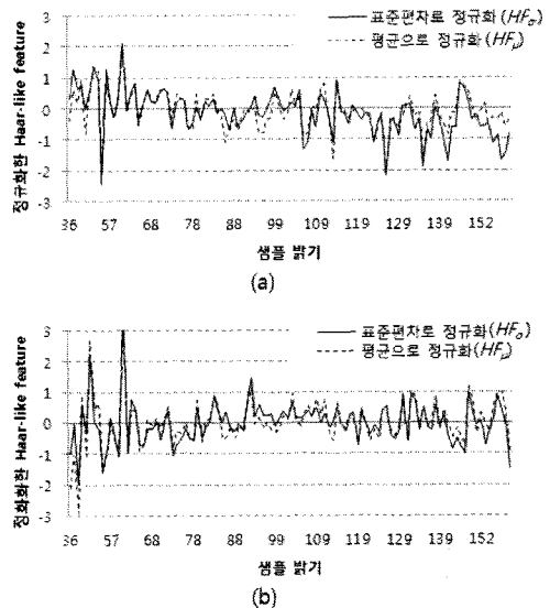
그림 7. 기존 방법과 제안한 방법으로 정규화한 Haar-like feature 값의 분포. (a) 첫 번째 Haar-like feature 값의 분포, (b) 두 번째 Haar-like feature 값의 분포
