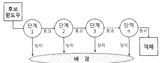
그림 3. 다단계 객체 분류기의 구성.
