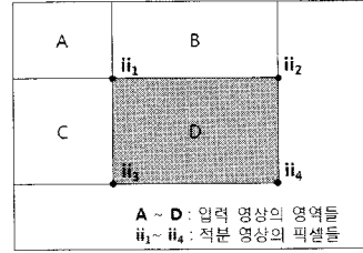
그림 2. 적분 영상을 이용한 사각형 영역 픽셀들의 합 계산. D 영역의 합은 ii_1 - ii_2 - ii_3 + ii_4 .
