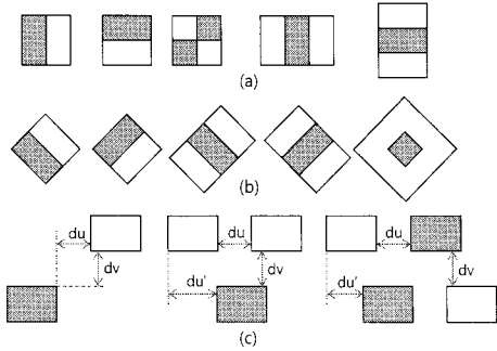
그림 1. Haar-like feature의 예. (a) Papageorgiou et al.의 Haar wavelet과 Viola와 Jones의 Haar-like feature, (b) Lienhart et. al의 45° 회전시킨 Haar-like feature, (c) Li et. al의 disjoint Haar-like feature.
