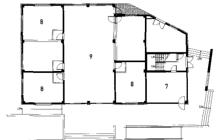
교육관/사제관 1층 평면도
