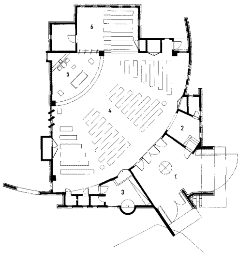
성당 1층 평면도
