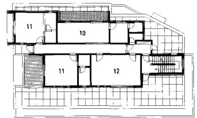
교육관/사제관 2층 평면도
