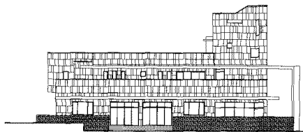
교육관/사제관 정면도
