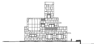
교육관/사제관 좌측면도
