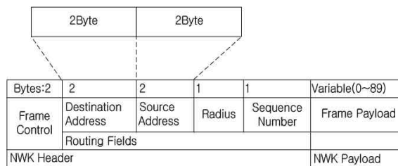
그림4. 네트워크 계층의 프레임 형식 Fig.4. The network layer frame format
