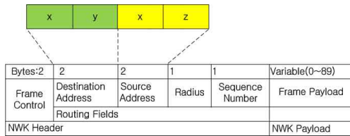
그림5. 제안하는 네트워크 계층의 프레임 형식 Fig.5. The network layer frame format of the proposed
