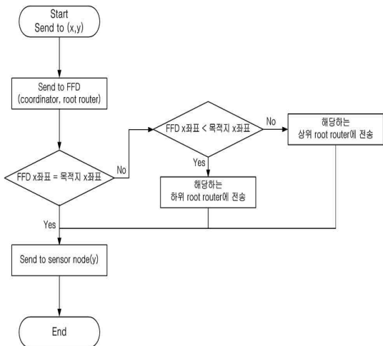
그림6. (x, y) 좌표 라우팅 흐름도 Fig.6. (x, y) coordinates routing Flow
