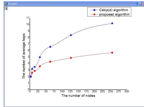
그림10. (4, 4) 좌표 총 255개 노드 Fig.10. (4, 4) coordinate the total node 255
