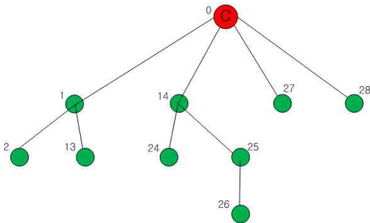
그림3. C_m = 4, R_m = 2, L_m = 3 일 때의 주소 할당 Fig.3. Address allocation when C_m = 4, R_m = 2, L_m = 3
