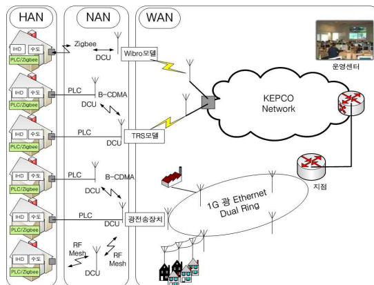
그림 1. 통신망 및 운영센터 구성도 Fig 1. Architecture of communications network and Operation Center architecture.
