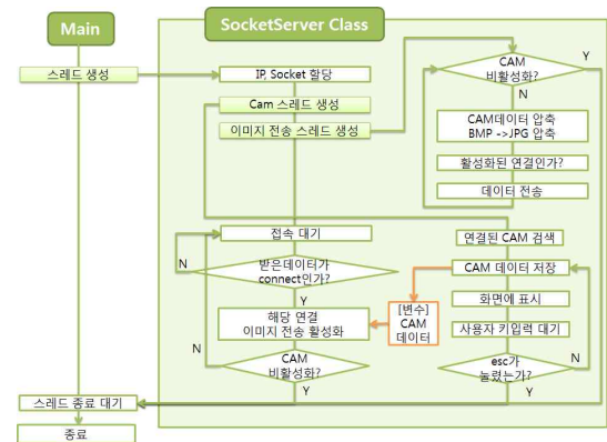
그림 2. 서버 흐름도 Fig. 2. Flowchart of a Server
