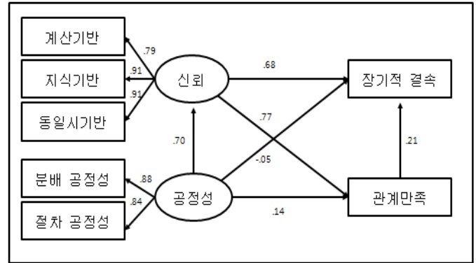
<그림 2> 경로분석 결과
