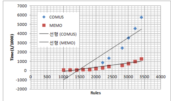
그림 11. COMUS와 MEMO에 대한 추론 시간 Fig. 11. Inference time of MEMO and COMUS
