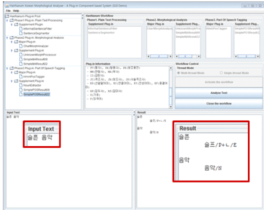
그림 6. Q1에 대한 형태소 분석 결과 Fig. 6. Morphological analysis of Q1 results
