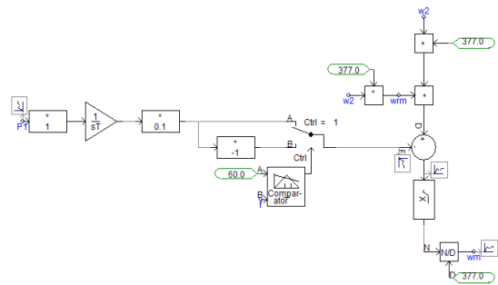
P_f: 플라이휠일의 출력전력 1/sT: 적분기
