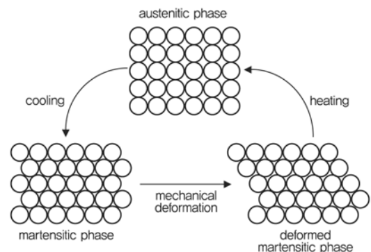
(그림 1) 형상기억합금의 형상기억 원리
