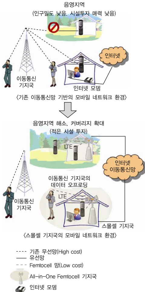
(그림 1) 통신망 내에서의 LTE 펠토셀 기지국 위치
