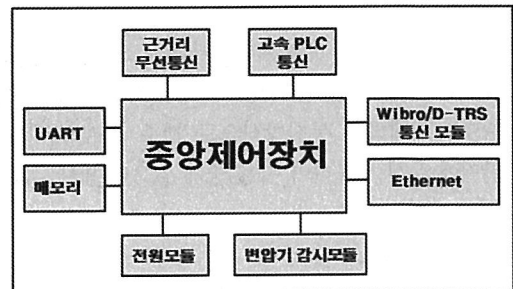
【그림 2】 데이터 전송장치의 HW 구성도
