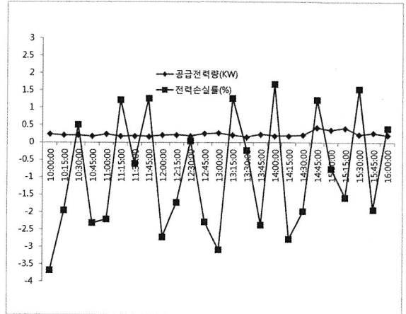
【그림 7】 전력손실률 그래프(평일)
