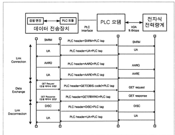
[그림 3] DLMS/COSEM 기반의 검침데이터 수집절차
