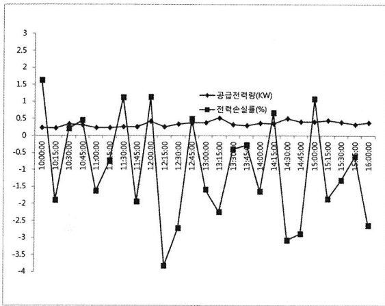
【그림 6】 전력손실률 그래프(주말)
