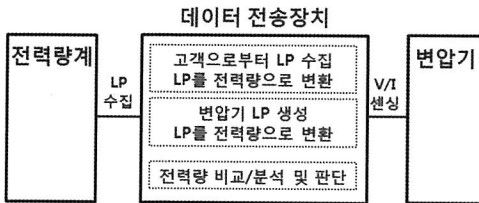
【그림 4】 데이터 전송장치의 전력량 산정방법
