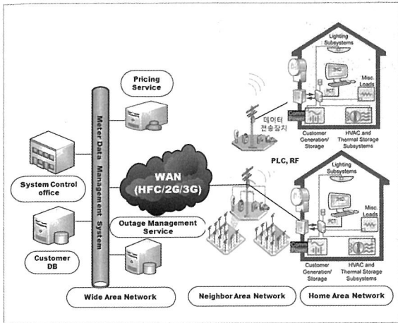
【그림 1】 지능형 원격검침 시스템 구성도
