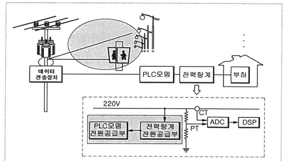
【그림 5】 데이터 전송장치에서 수집 불가능한 전력 사용량
