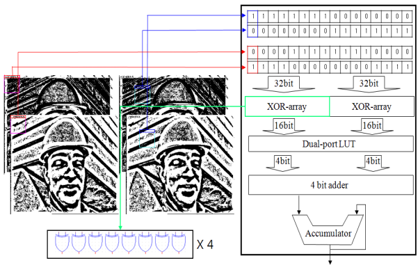
그림 4. 제안한 방법의 R-SAD 2-bit 의 하드웨어 구조 Fig. 4. Hardware structure for calculating R-SAD 2-bit in proposed method.
