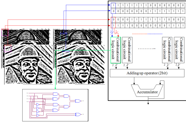
그림 3. 2BT의 NNMP를 계산하는 하드웨어 구조. Fig. 3. Hardware structure for calculating NNMP in 2BT.
