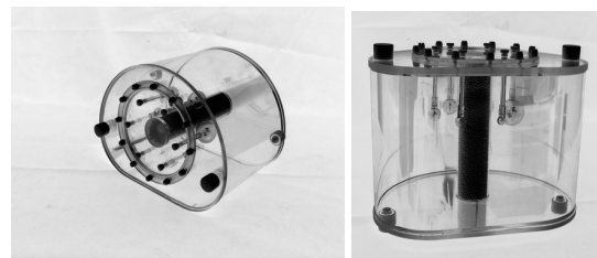
Fig. 1. NEMA IEC Body Phantom
