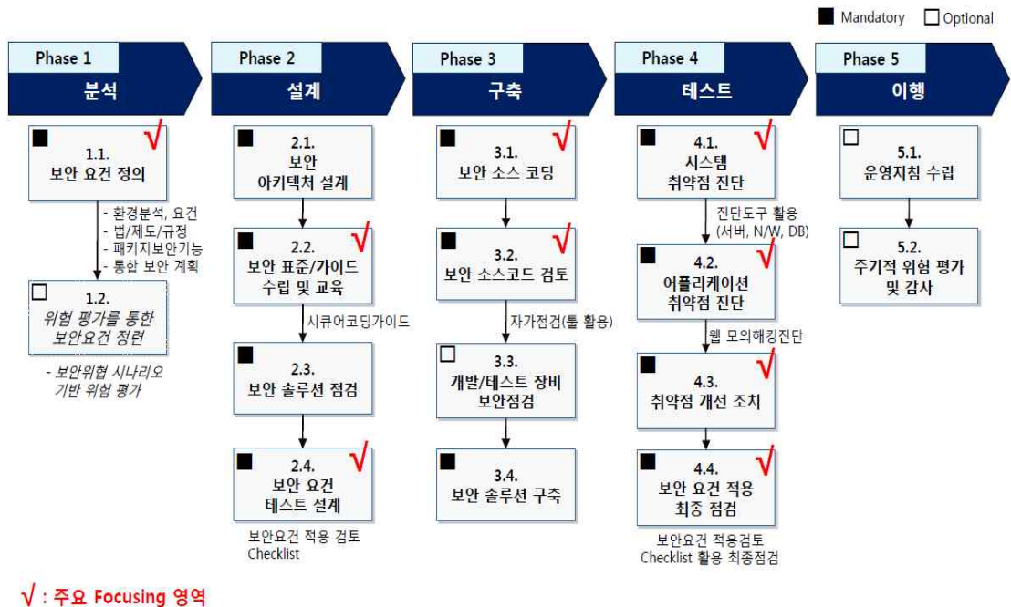
그림 1. 단계별 주요 보안 Activity Fig. 1. Step-Wide Security Activity
