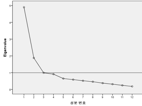
<그림 1> 도서관 인식 요인분석: 스크리 도표
