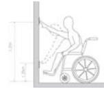
각종 스위치 및 인터폰 사용 : 휠체어 사용자 도달 범위 (높이 35-120cm 범위에 설치)
