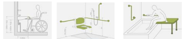
휠체어사용자의 세면대 이용 : 세면대 하부공간 확보 샤워공간 접의식의자, 수평손잡이, 높낮이 조절형 샤워기 설치 휠체어 사용자의 욕조이용 : 욕조의 높이, 휠체어 및 이동의자 높이 (40-45cm)
