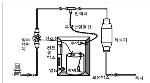
▲ 자동투약장치 모식도(좌)와 설치된 모습(우)
