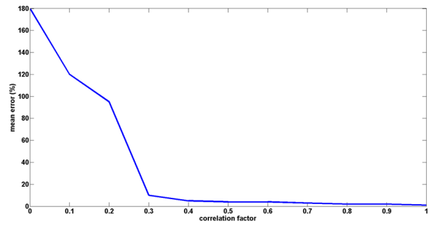
그림 7. 상관인수에 따른 속도 추정 오차 Fig. 7. Error of estimated velocity with respect to correlation factor.
