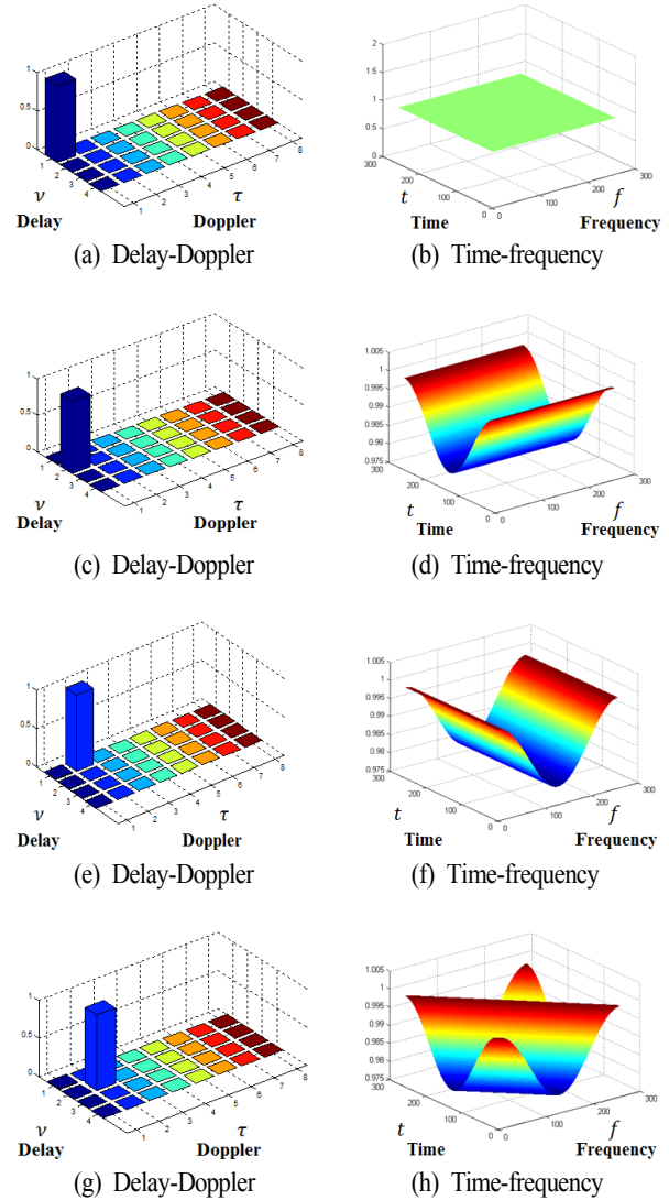
그림 3. OTFS 기저 함수 Fig. 3. OTFS basis function.
