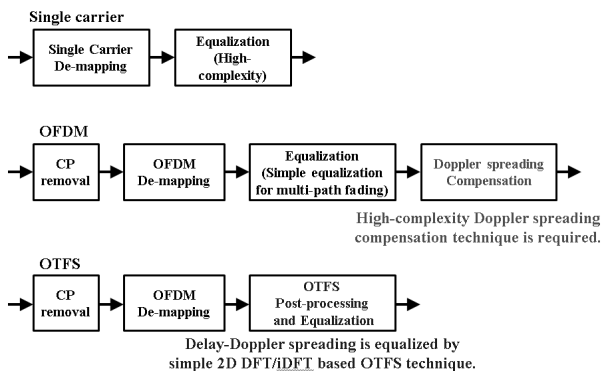
그림 2. 단일 반송파, OFDM, OTFS의 수신기 구성도 Fig. 2. Receiver block diagram of single carrier, OFDM, OTFS.
