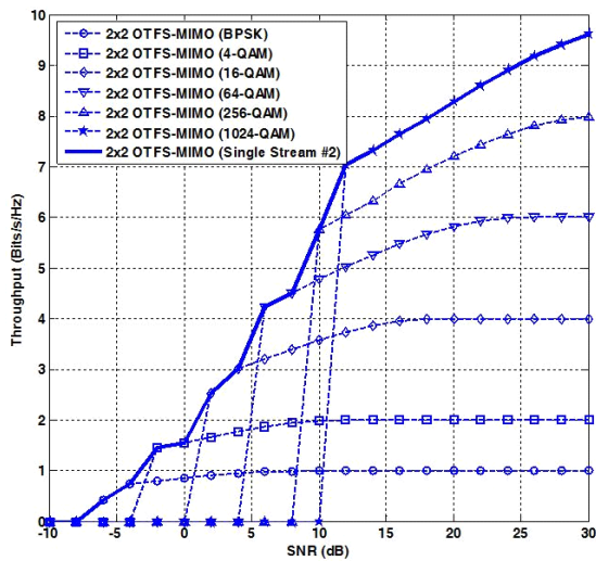
그림 13. 2x2 OTFS-MIMO(2번 스트림)의 전송률 Fig. 13. Achievable rate of 2x2 OTFS-MIMO(Stream #2).
