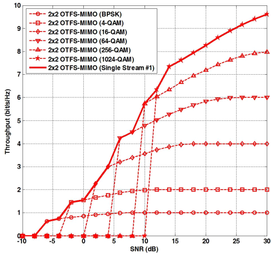
그림 12. 2x2 OTFS-MIMO(1번 스트림)의 전송률 Fig. 12. Achievable rate of 2x2 OTFS-MIMO(Stream #1).
