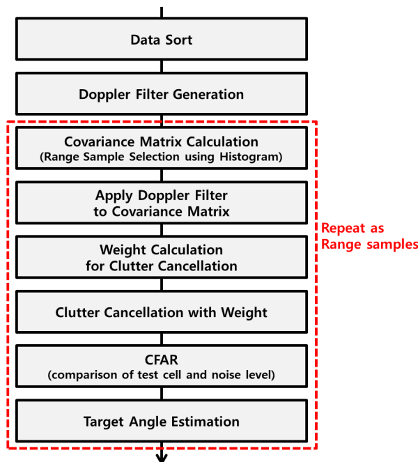
그림 3. STAP, CFAR, 각도 계산 상세 순서도 Fig. 3. Detailed flowchart for STAP, CFAR, angle estimation.
