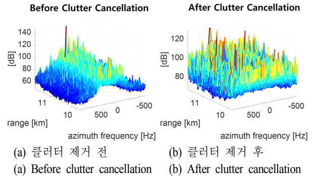
그림 7. 클러터 제거 전/후 거리-도플러 맵
