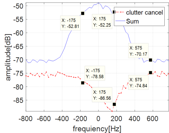
그림 8. 클러터 제거 성능
