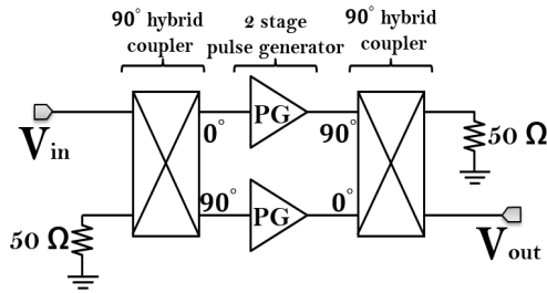
그림 2. 90° 하이브리드 커플러를 이용한 평형구조 기반 펄스 발생기
