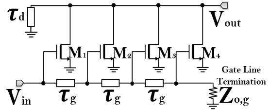
(a) 기존의 4단 구조 [2] (a) Conventional 4 stage structure
