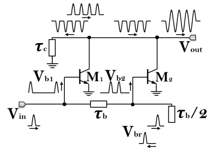
(b) 본 논문에서 사용한 2단 구조 (b) 2 stage structure in this work
