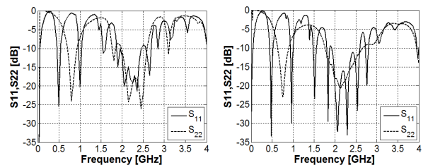
(d) S_{11}/S_{22} (시뮬레이션) (e) S_{11}/S_{22} (측정) (d) S_{11}/S_{22} (simulation) (e) S_{11}/S_{22} (measurement)
