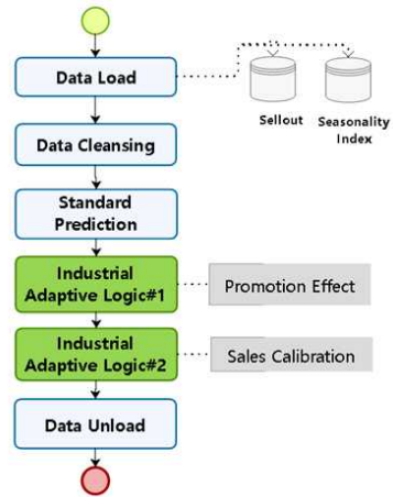
그림 9. 분석모델 프로세스 다이어그램 Fig. 9. Process Diagram of Model
