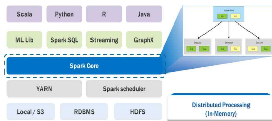
그림 6. 스파크 아키텍처 Fig. 6. Architecture of Spark
