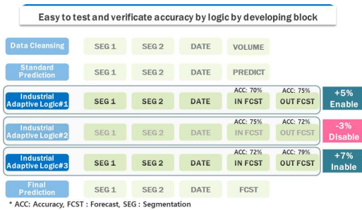
그림 8. 독립적인 로직 구현 및 검증 Fig. 8. Independent logic implementation/validation
