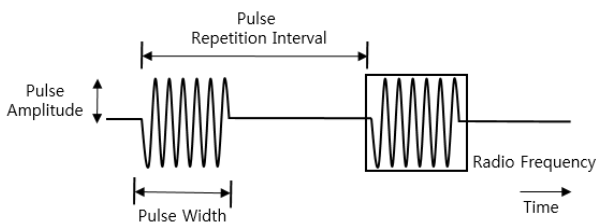
그림 1. 일반적인 펄스 레이더 신호 Fig. 1. Typical pulse radar signals.
