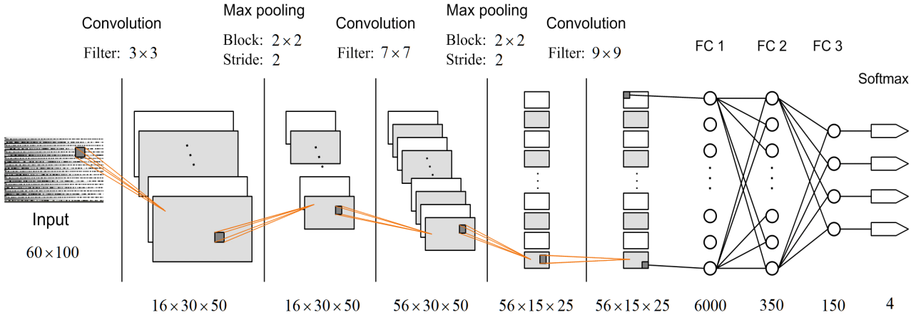
그림 10. CNN 구조 Fig. 10. Structure of the CNN.
