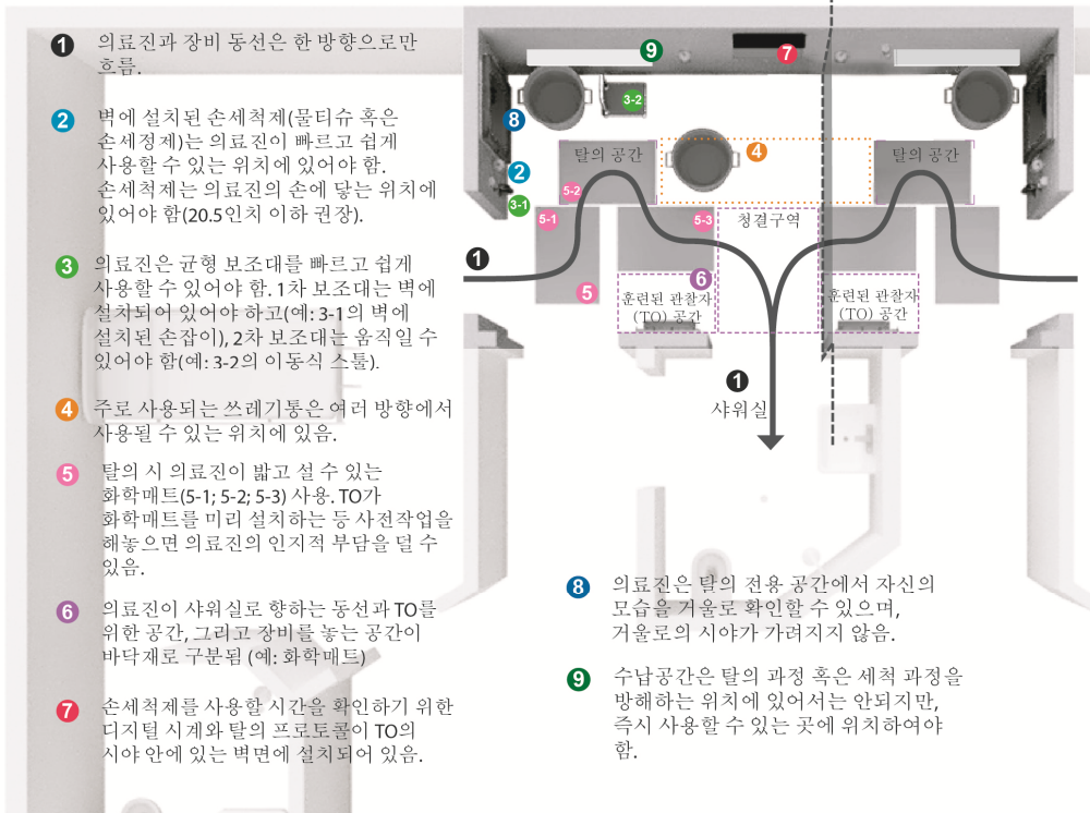
[그림 2] BCU 내 필요 장비들이 구분된 탈의 공간 레이아웃
