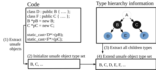
(그림 3) 객체 추적 최적화 방법 개요
