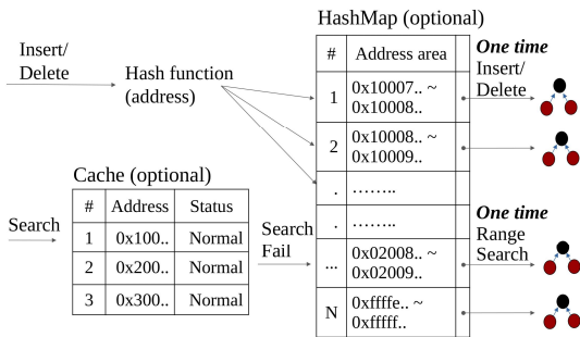
[그림 5] RB-tree 메타데이터 구조
