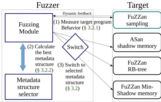
[그림 4] FuZZan 프로젝트 개요
