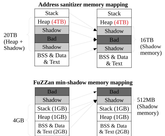
[그림 6] Min-shadow 메타데이터 구조
