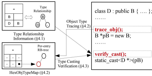
(그림 1) HexType 프로젝트 개요
